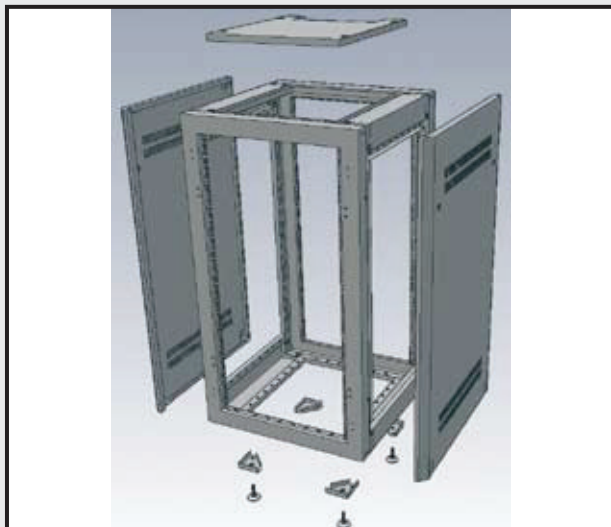
Gestellschrank mit Zubehör
